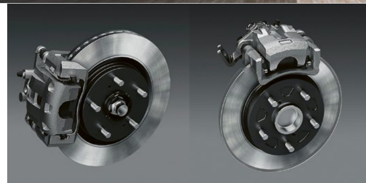
Disques ventilés de 16 pouces à l'avant.
